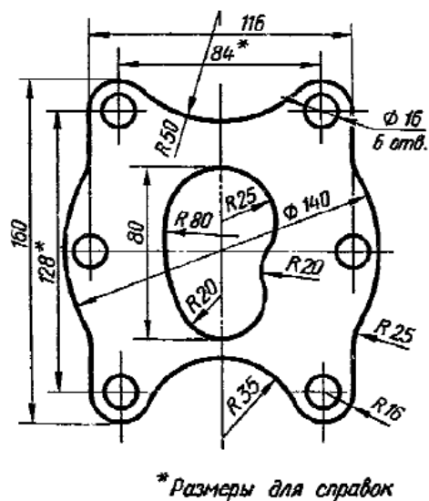
Чертёж 2
