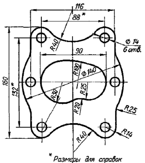
Чертёж 1
