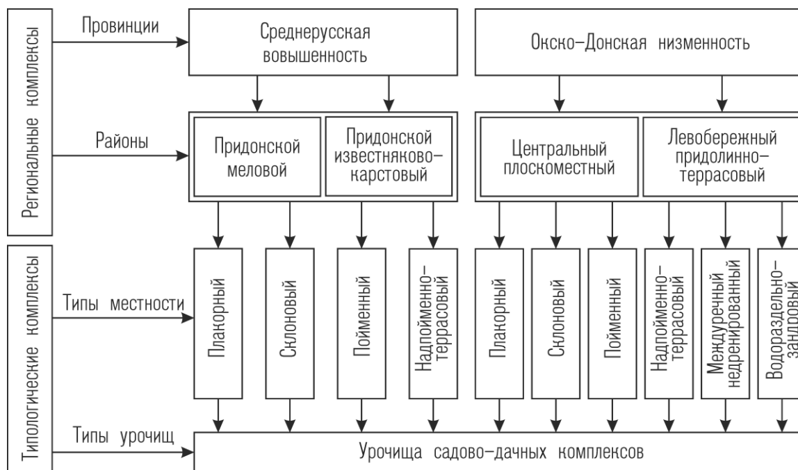
Рис. 33. Место СДК в системе ландшафтных комплексов Подворонежья
