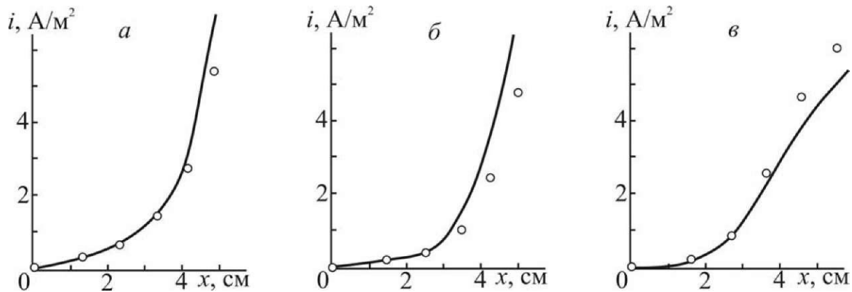
Рис. 3.10. Функция распределения скорости коррозии вдоль железной пластины при линейном (а), экспоненциальном (б) и параболическом (в) распределении температуры. Точки — экспериментальные значения. Условия эксперимента — как на рис. 3.9
