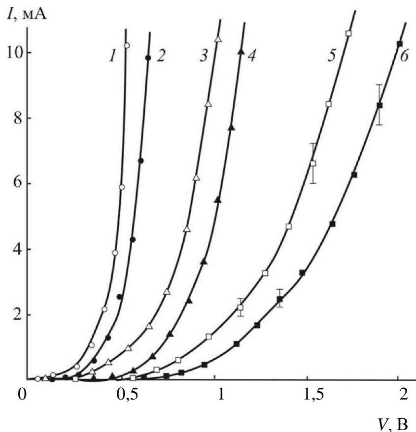
Рис. 1.1. Вольт-амперные характеристики р-п-переходов из германия (1, 2), кремния (3, 4) и арсенида галлия (5, 6) при температуре 20 (2, 4), 80 (1), 100 (3, 6) и 150 (5) °С (рисунок заимствован из [12])
