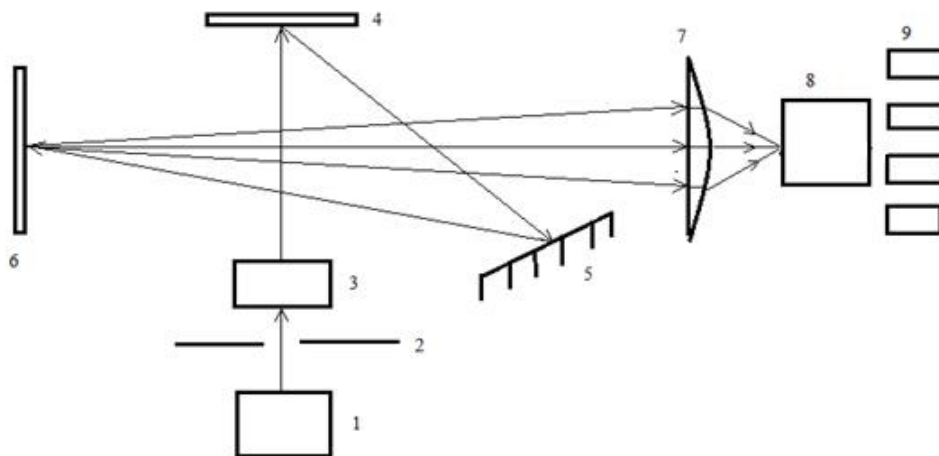
1 – оптический разъём SMA 905; 2 – щель; 3 – фильтр; 4 – коллимирующее зеркало; 5 - дифракционная решётка; 6 – фокусирующее зеркало; 7 – собирающая линза; 8 – детектор; 9 – линейные перестраиваемые фильтры (опция)
