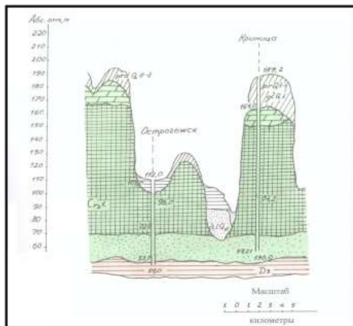
Рисунок 2 - Геологический разрез по линии Острогжск-Креница [ссылка на источник дается по его номеру в списке литературы]
