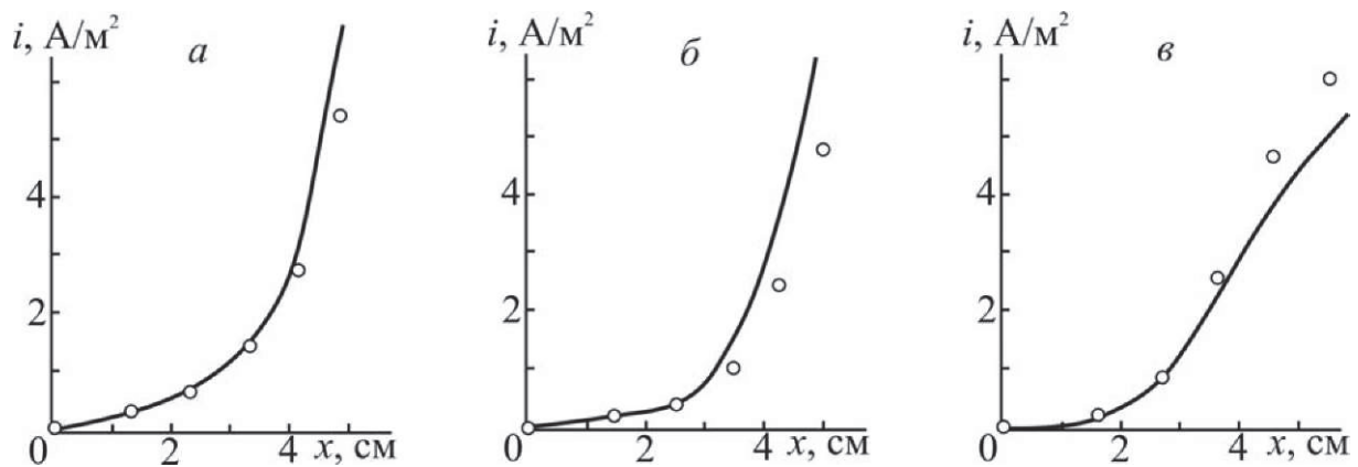
Рис. 3.10. Функция распределения скорости коррозии вдоль железной пластины при линейном (а), экспоненциальном (б) и параболическом (в) распределении температуры. Точки – экспериментальные значения.
