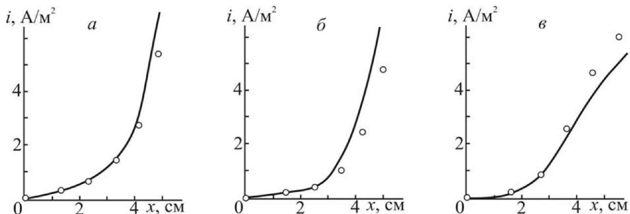
Рис. 3.10. Функция распределения скорости коррозии вдоль железной пластины при линейном ( a ), экспоненциальном ( б ) и параболическом ( в ) распределении температуры. Точки — экспериментальные значения. Условия эксперимента — как на рис. 3.9
