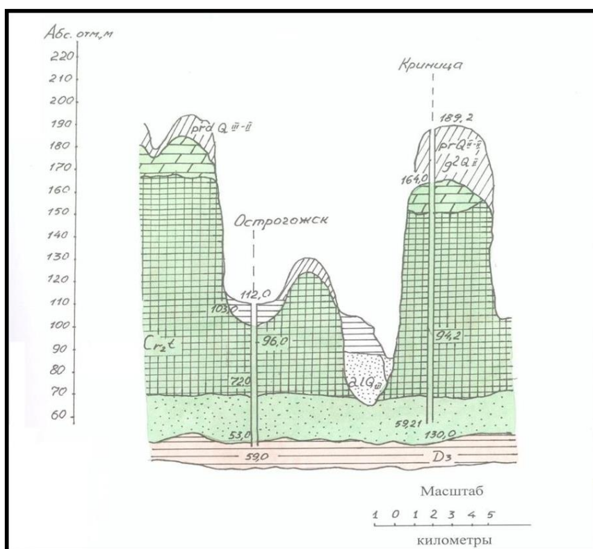
Рисунок 2 - Геологический разрез по линии Острогжск-Крымцига [ссылка на источник дается по его номеру в списке литературы]
