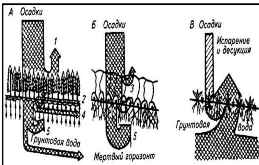
1 – испарение с растительной поверхности; 2 – поверхностный сток; 3 – испарение с поверхности почвы; 4 – внутрипочвенный сток; 5 – десукция.
